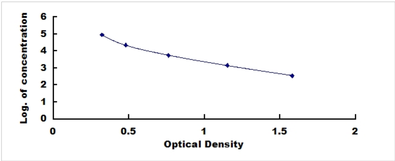
雄甾酮 (ADT) 检测试剂盒标准曲线
