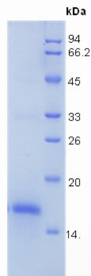
15% SDS-PAGE
