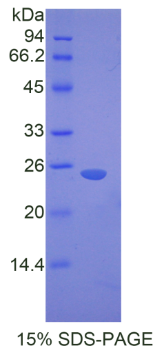
15% SDS-PAGE
