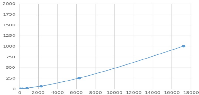
(10kDa干扰素 \gamma 诱导蛋白)检测试剂盒标准曲线
