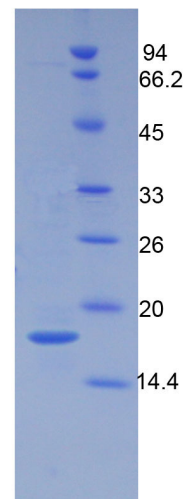
15% SDS-PAGE
