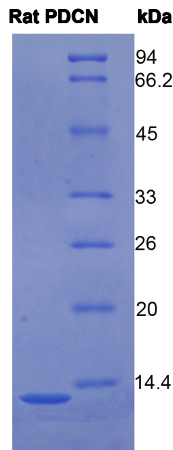
15% SDS-PAGE
