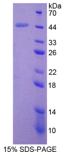
15% SDS-PAGE
