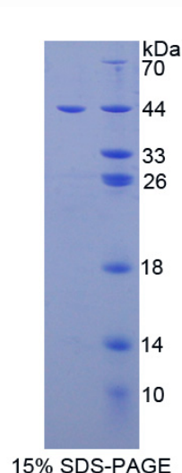
15% SDS-PAGE
