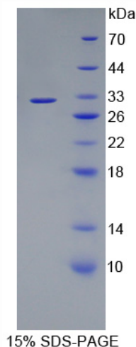
15% SDS-PAGE
